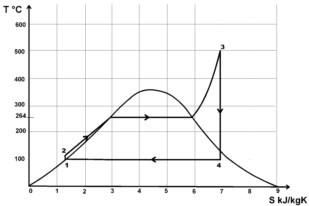
Diagrama T-s
